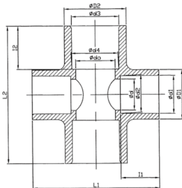
異徑十字通
