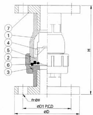
VP-460 F
