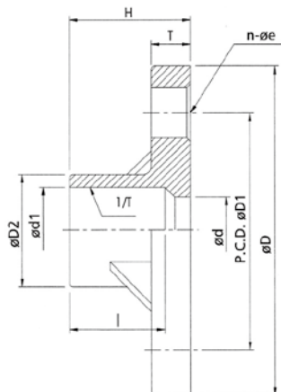
JIS 10K
